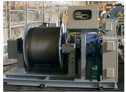
光スリップリング仕様検層用ウインチ
